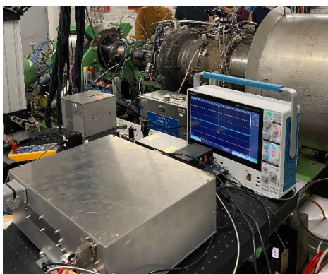
Figure 1. Allumeur laser sur moteur Safran-HE.
